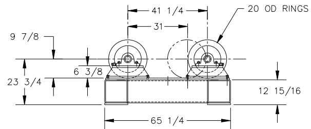
VIEW A-A
